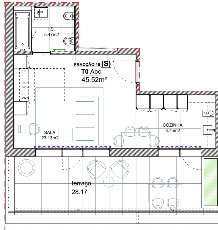
PLANTA 1/100
