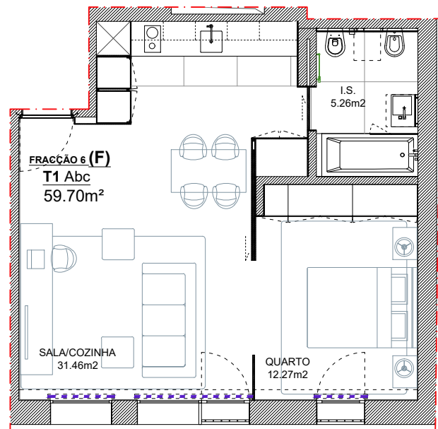
PLANTA 1/100
