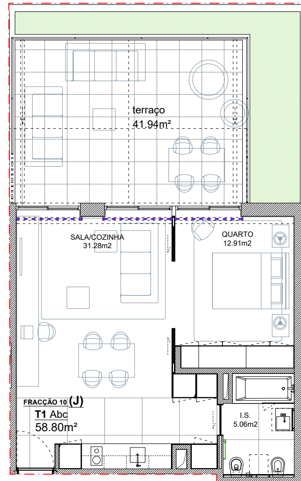
PLANTA 1/100
