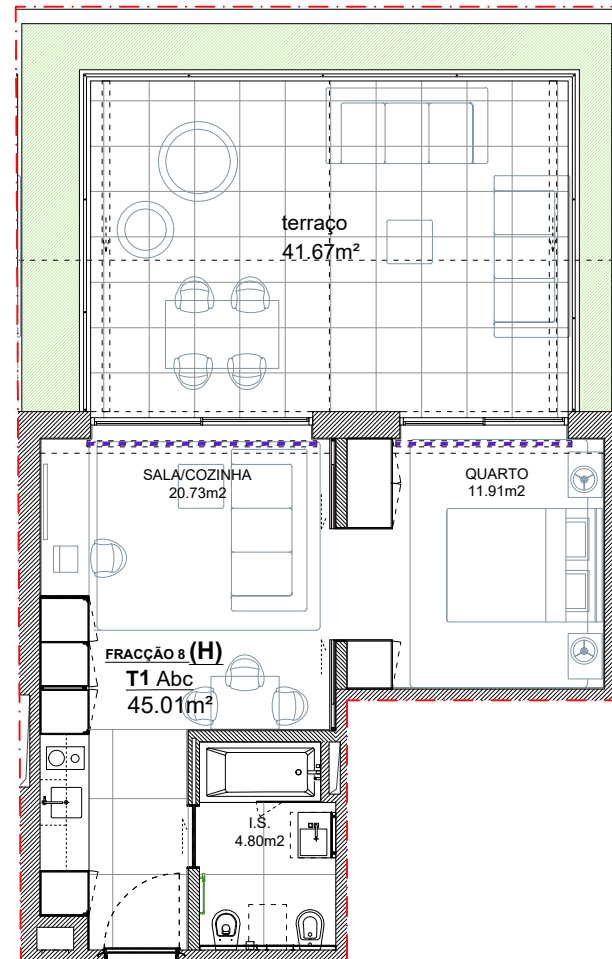
PLANTA 1/100
