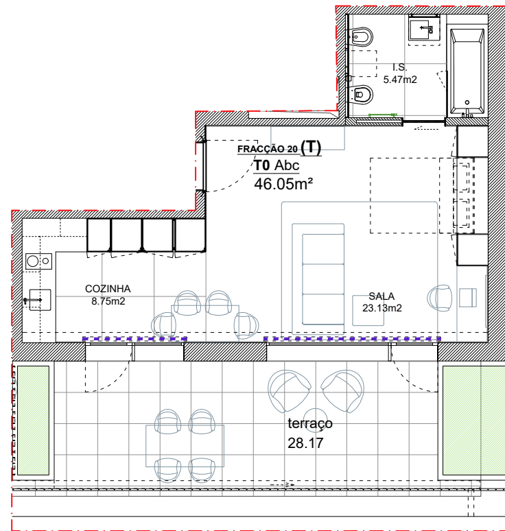
PLANTA 1/100
