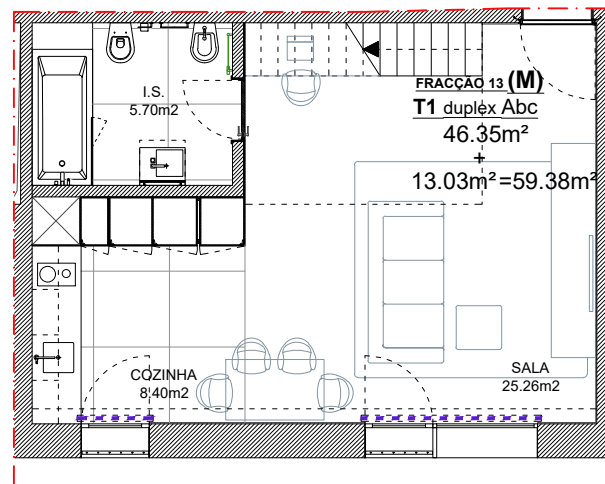
PLANTA (2º PISO) 1/100
