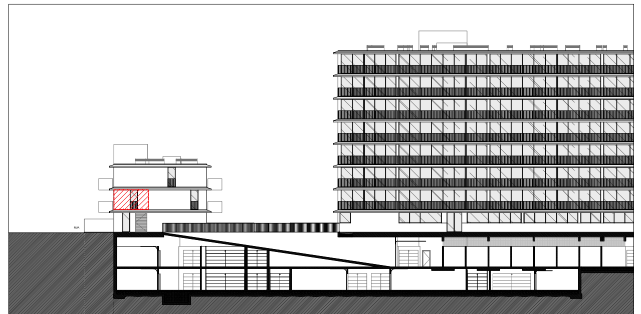
ALÇADO/ CORTE 5 1/500
