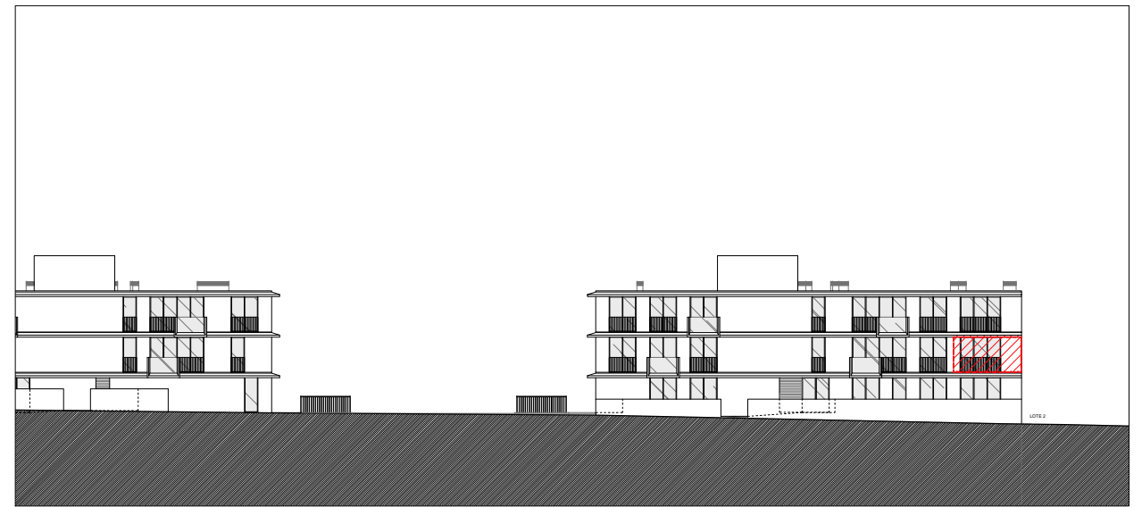
ALÇADO NORTE 1/500
