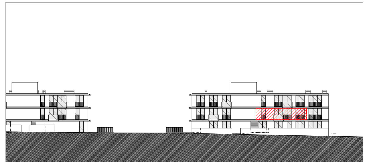
ALÇADO NORTE 1/500
