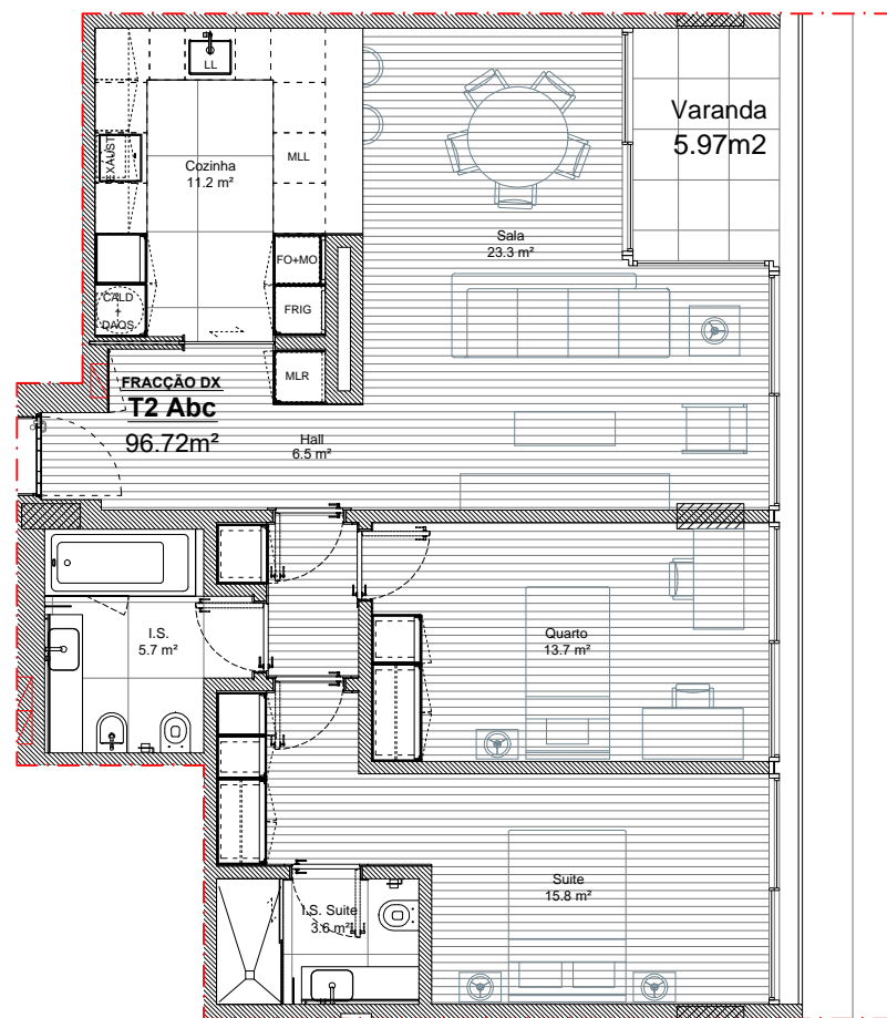
PLANTA 1/100
