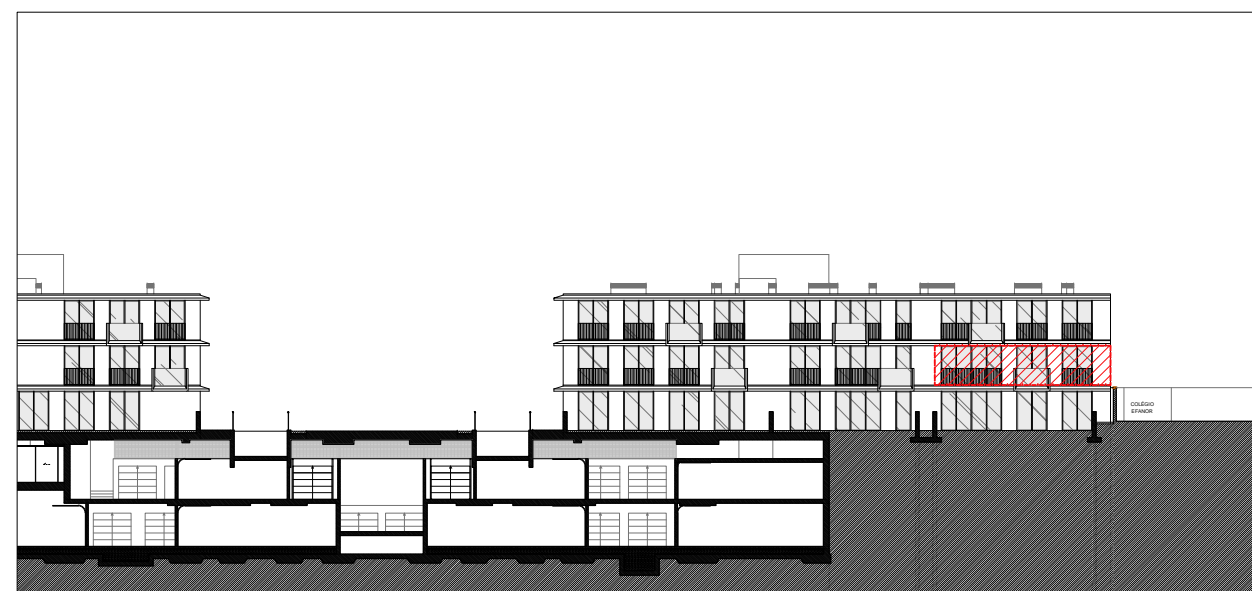
ALÇADO/ CORTE 8 1/500
