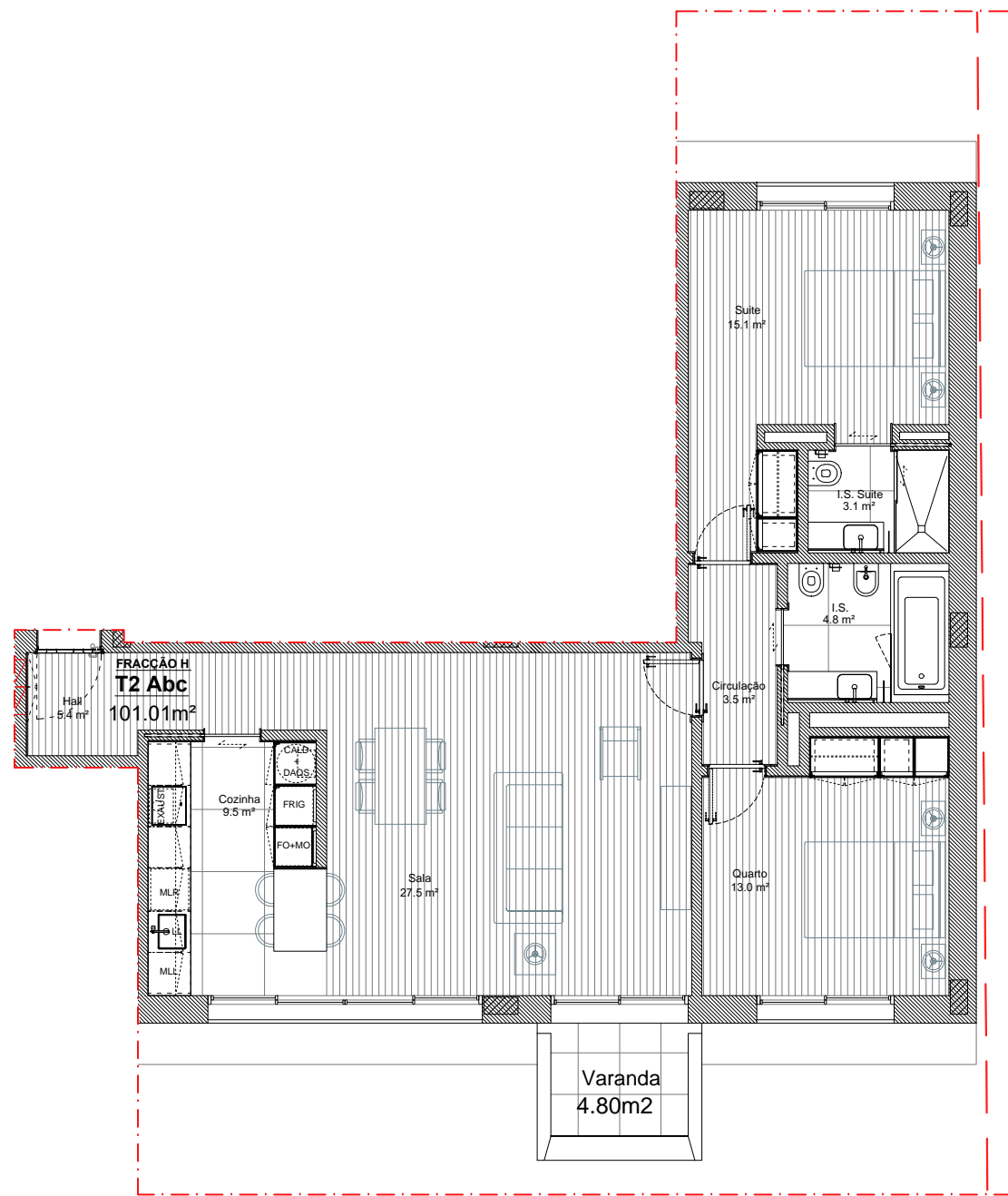
PLANTA 1/100
