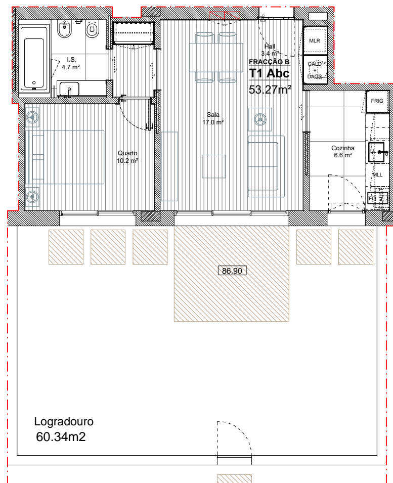
PLANTA 1/100
